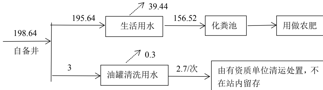
图 5 项目水量平衡图 (m 3 /a)
