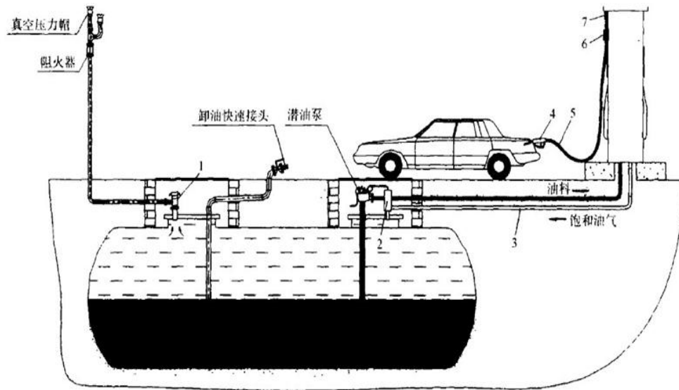
1—油气回收快速接头;2—真空泵;3—油气回收管;4—油气回收油枪;5—同轴胶管;6—胶管脱离器;7—油气分离转换接头
